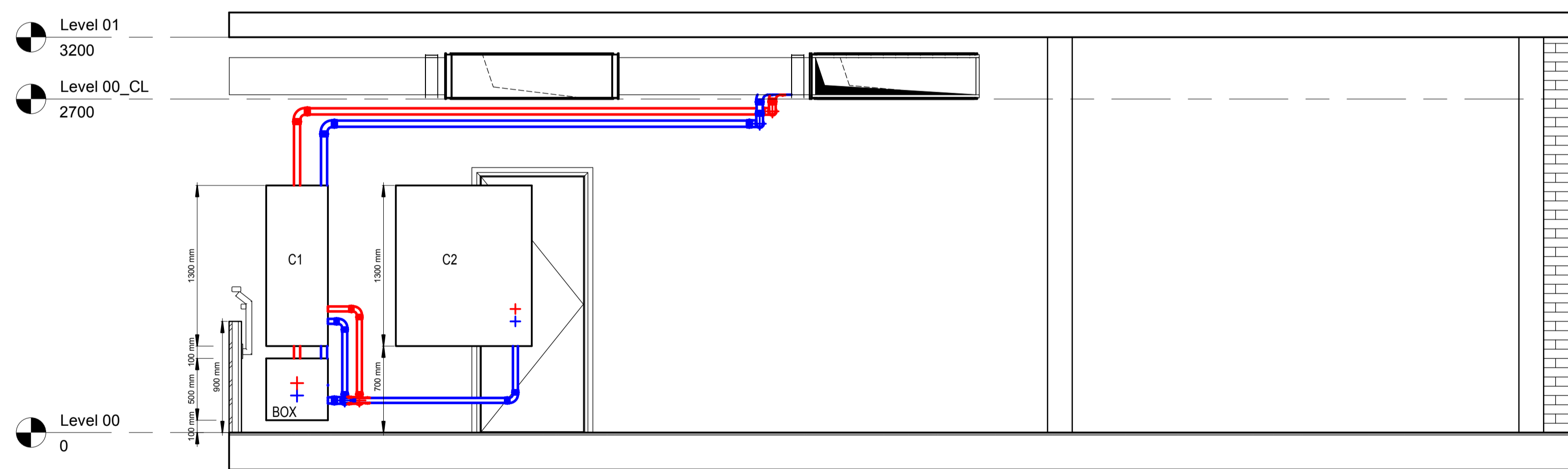
3 Detail 2 1 : 30
