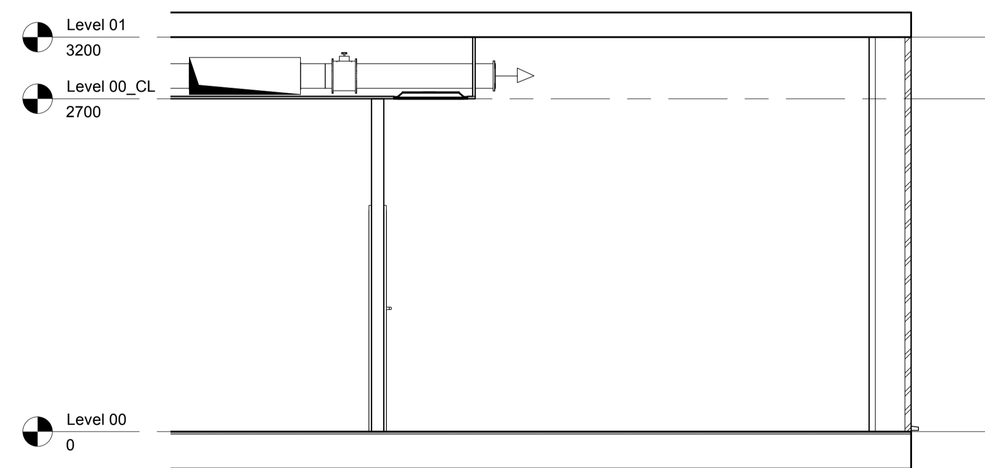
2 Detail 3 1 : 30
